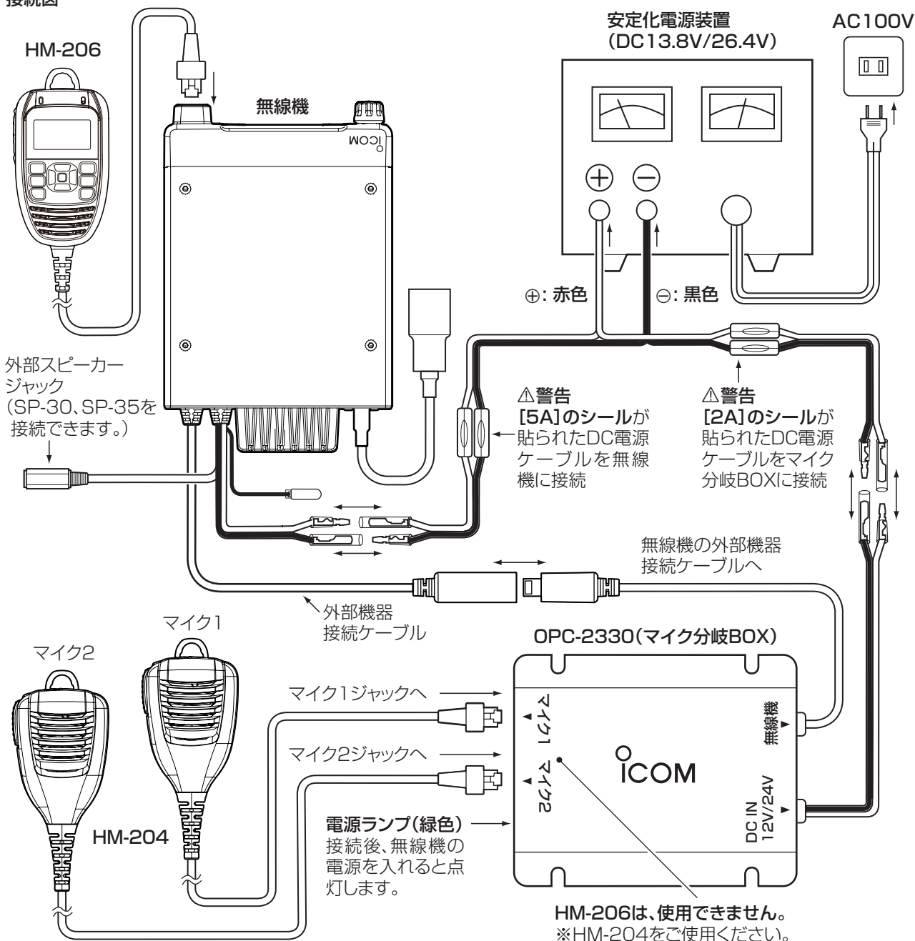
接続図
